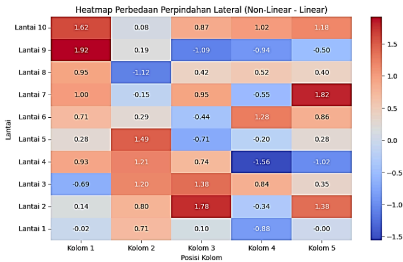
Gambar 1. Distribusi Perpindahan Lateral pada Struktur
