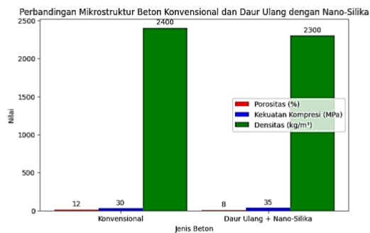
Gambar 2. SEM Perbandingan Mikrostruktur
