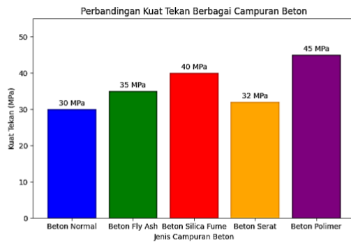
Gambar 1. Perbandingan Kuat Tekan
